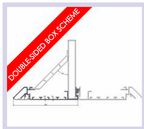
AL podpora ID VYNILPODP125T1,74P1142 Aluminium bracket for 125 mm profile - 0,75 Euro/pcs
